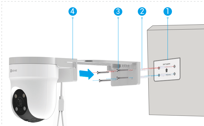
Hình 2 Gắn tường
