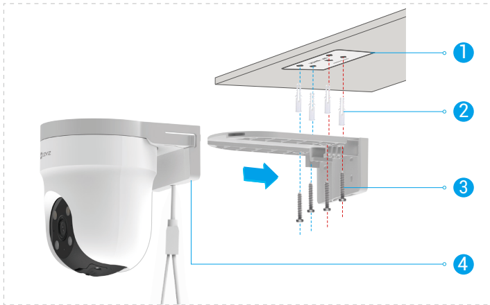
Hình 1 Gắn trần
